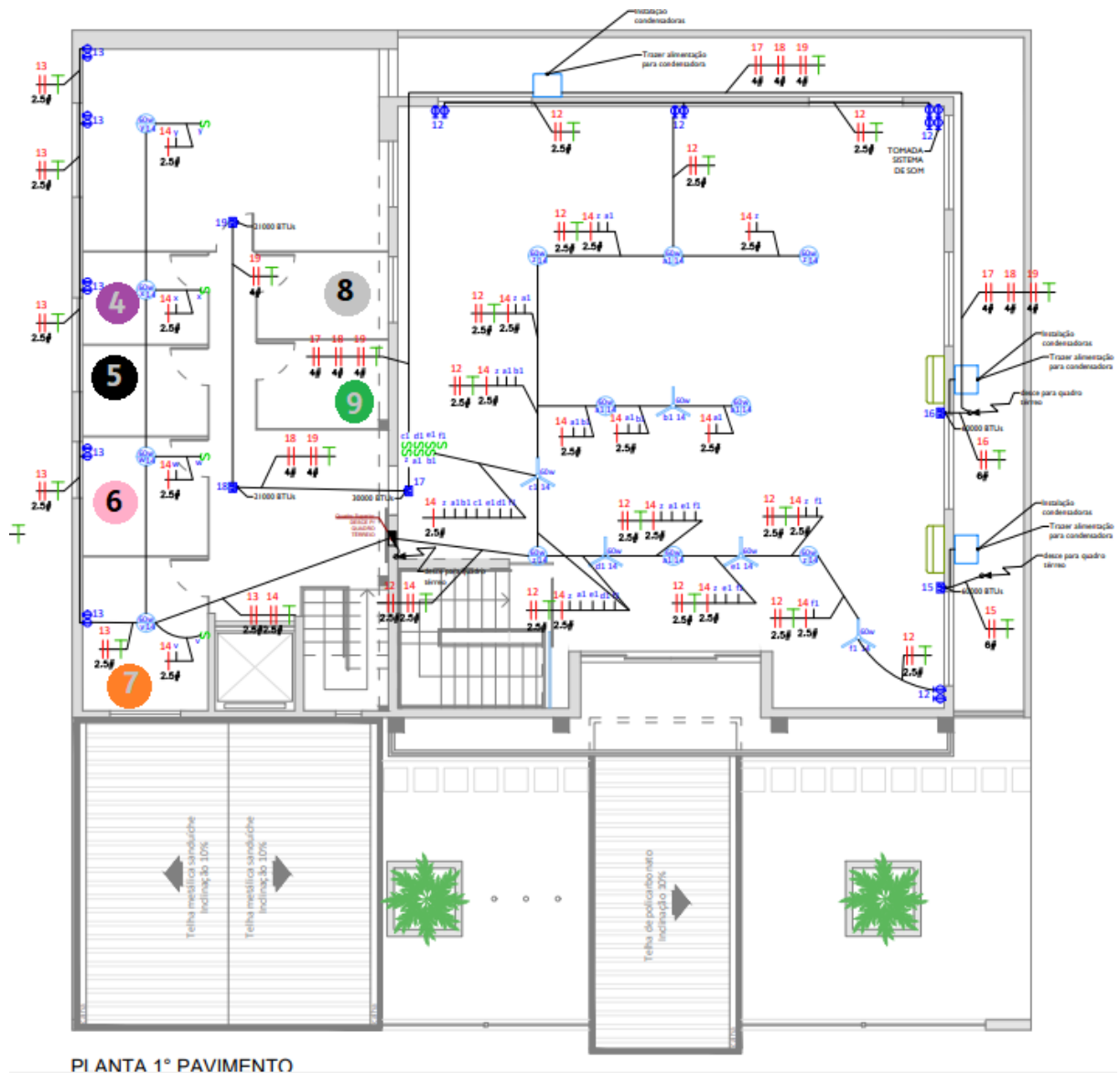
Figura 3: Instalações do 1º pavimento
